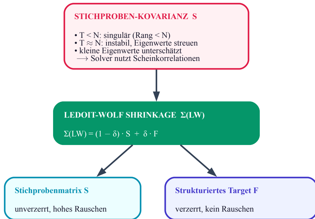
Abbildung 38: Abb. 18.1: Ledoit-Wolf-Kovarianz-Shrinkage
