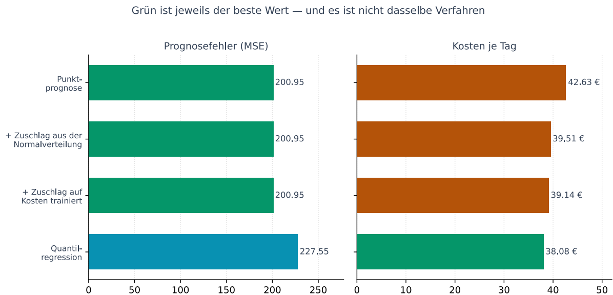
Abbildung 35: Abb. 15.1: Dieselben vier Verfahren, zwei Maßstäbe. Grün ist jeweils der beste Wert. Erzeugt von bilder_04/erzeuge_predict_vs_optimize.py .
