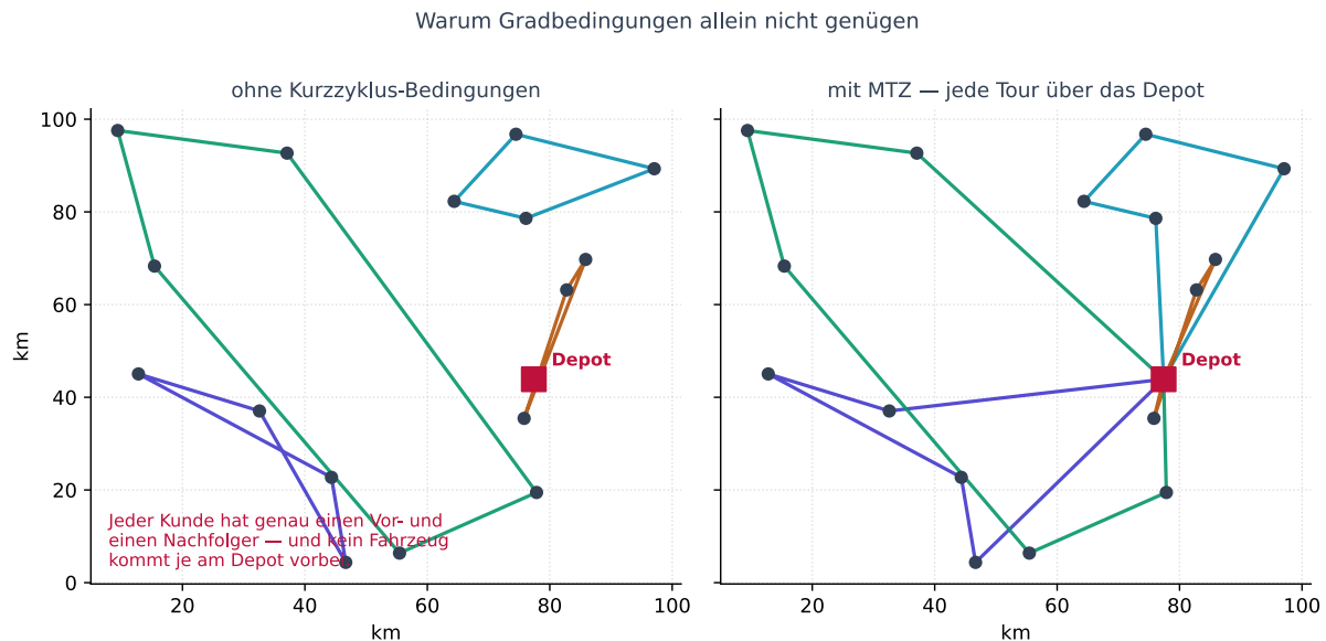
Abbildung 25: Abb. 8.3: Links eine Lösung, die jede Gradbedingung erfüllt und trotzdem unbrauchbar ist; rechts dieselbe Instanz mit Kurzzyklus-Bedingungen. Erzeugt von bilder_04/erzeuge_vrp_subtours.py .
