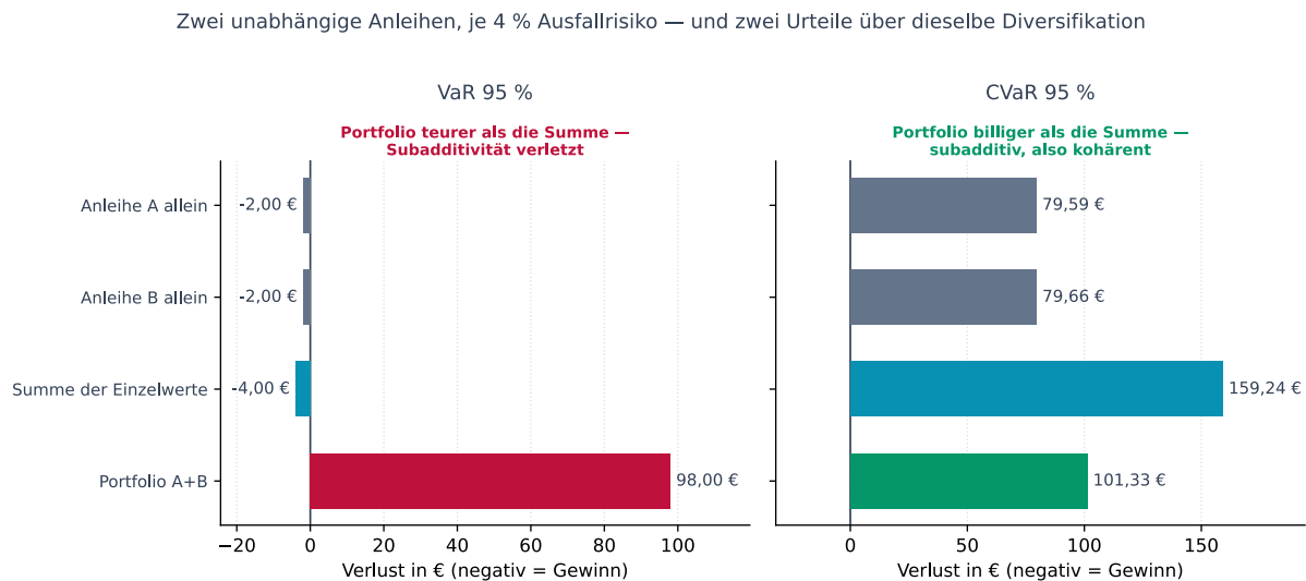
Abbildung 41: Abb. 20.1: Dieselbe Tabelle als Bild, gerechnet mit denselben Ziehungen wie VaR_CVaR_Demo.py. Erzeugt von bilder_04/erzeuge_var_vs_cvar.py.
