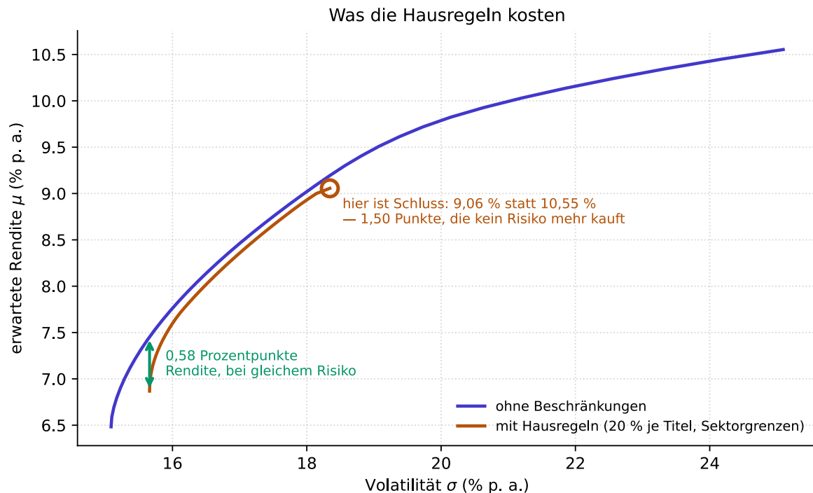
Abbildung 40: Abb. 19.2: Was die Hausregeln kosten. Der senkrechte Abstand ist der Renditeverlust bei gleichem Risiko. Wichtiger ist aber das rechte Ende: Mit den Hausregeln bricht die Linie bei 9,06 % ab — die letzten 1,50 Punkte sind mit keinem Risiko der Welt mehr zu kaufen. Feste Instanz aus einem Faktormodell, erzeugt von bilder_04/erzeuge_effizienzlinie.py .
