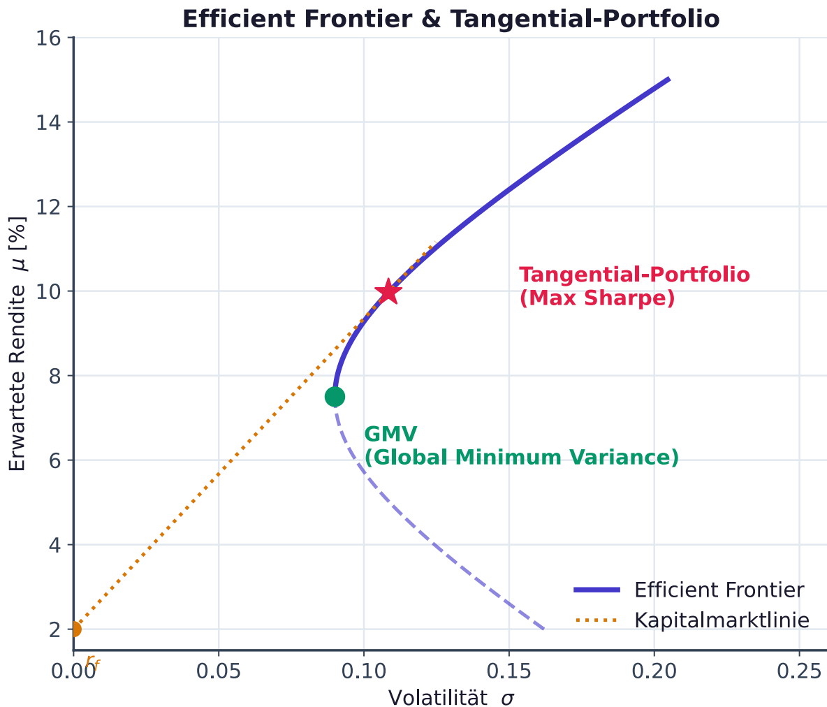
Abbildung 39: Abb. 19.1: Efficient Frontier und Tangential-Portfolio
