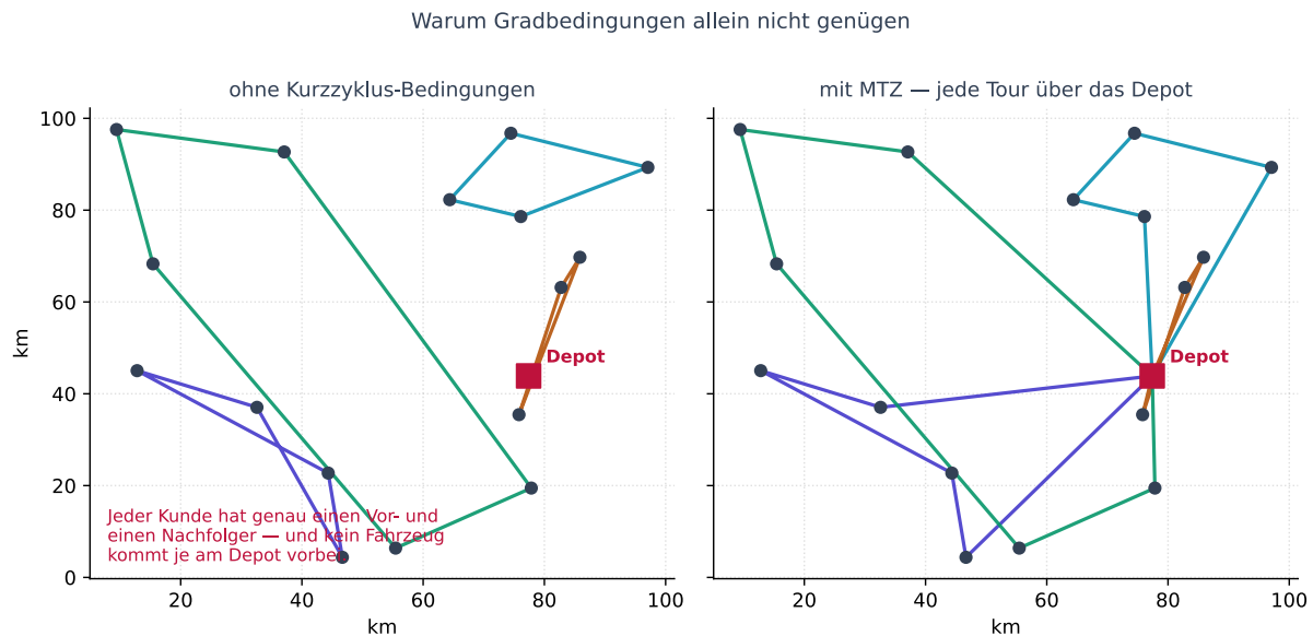
Abbildung 25: Abb. 8.3: Links eine Lösung, die jede Gradbedingung erfüllt und trotzdem unbrauchbar ist; rechts dieselbe Instanz mit Kurzzyklus-Bedingungen. Erzeugt von bilder_04/erzeuge_vrp_subtours.py .
