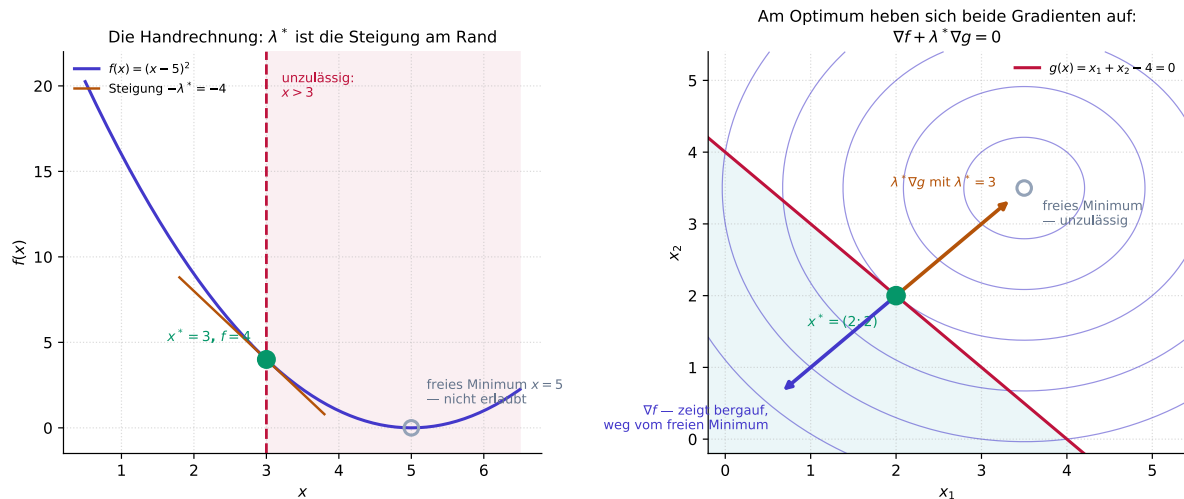
Abbildung 18: Abb. 11.1: Links die Handrechnung dieses Abschnitts: Das freie Minimum liegt bei x = 5 , die Grenze lässt nur x \leq 3 zu, und \lambda^* = 4 ist genau die Steigung von f am Rand — der Preis dafür, dass es nicht weitergeht. Rechts dieselbe Aussage in zwei Dimensionen: \nabla f und \lambda^* \nabla g zeigen gegeneinander und heben sich auf. Das Skript bilder_04/erzeuge_kkt.py prüft alle vier KKT-Bedingungen numerisch, bevor es zeichnet.
