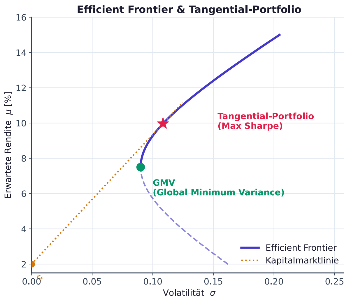
Abbildung 24: Abb. 19.1: Efficient Frontier und Tangential-Portfolio
