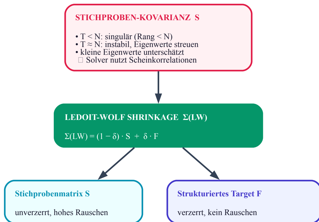
Abbildung 22: Abb. 18.1: Ledoit-Wolf-Kovarianz-Shrinkage
