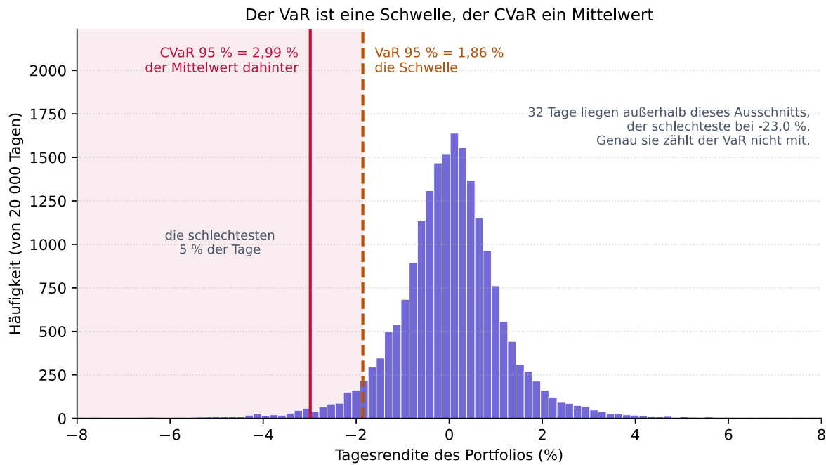
Abbildung 25: Abb. 20.1: Der VaR ist eine Schwelle, der CVaR ein Mittelwert. 20 000 simulierte Tagesrenditen aus dem Fat-Tail-Modell dieses Kapitels ( t -Verteilung mit drei Freiheitsgraden). Der schraffierte Bereich sind die schlechtesten 5 % der Tage; der VaR markiert nur ihren Rand, der CVaR ihren Mittelwert. Erzeugt von bilder_04/erzeuge_var_cvar.py .
